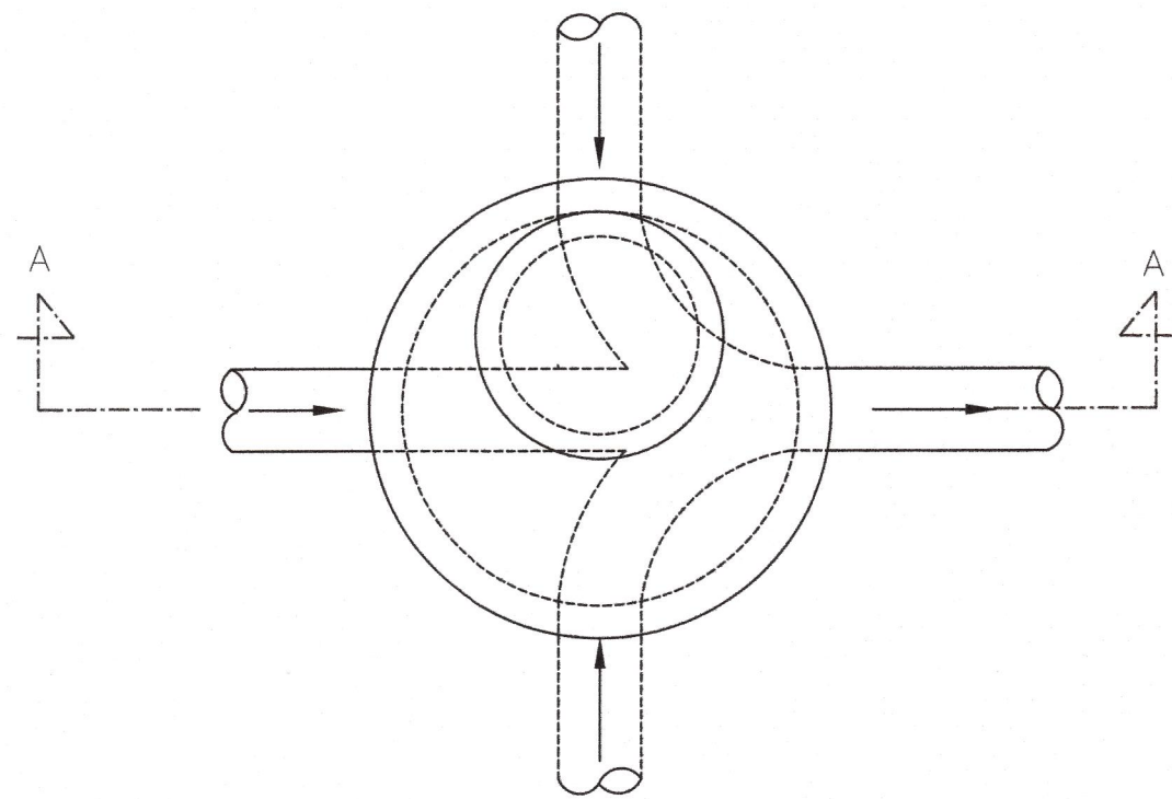
PLANTA
